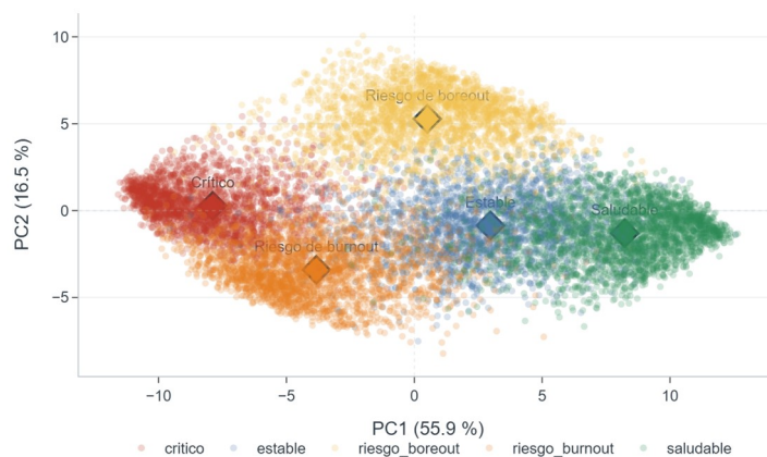
Figura 2. Proyección del benchmark sobre las dos primeras componentes principales (PCA).
